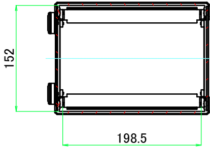
B-B ( 1 : 5.5 )
