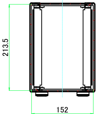
A-A ( 1 : 5.5 )
