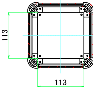
C-C ( 1 : 5.5 )
